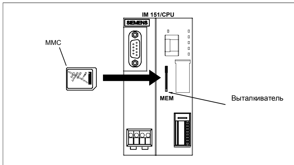
Рисунок 5-3 Позиция слота карточки памяти для MMC на IM 151/CPU
