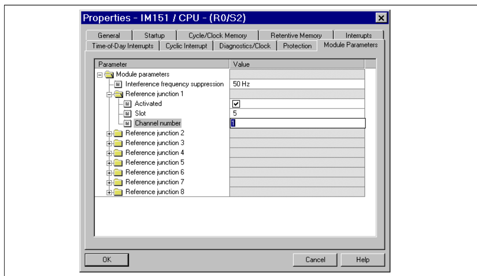
Рисунок 5-4 Пример параметризации диалогового окна для данных модуля CPU в STEP 7 V5.1
