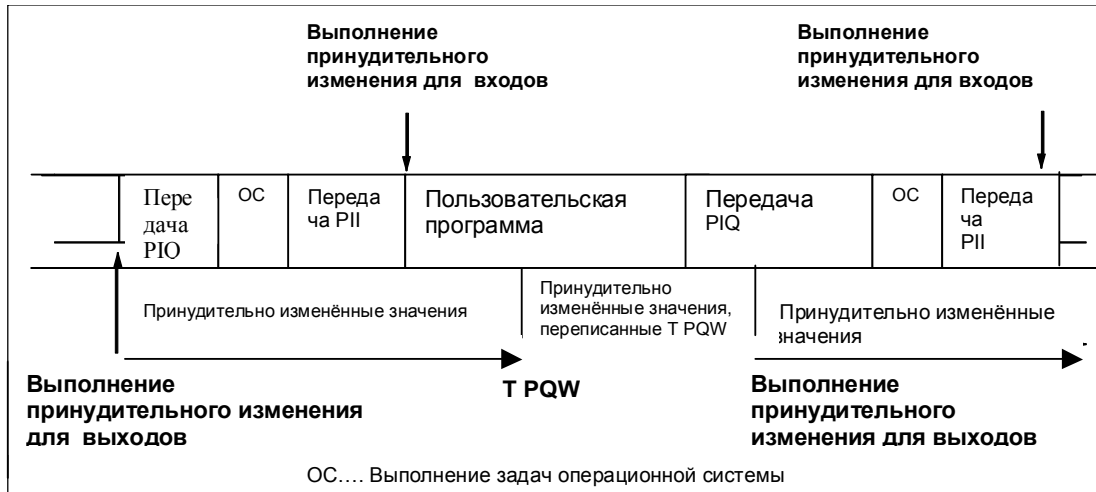
Рисунок 5-2 Принцип принудительного изменения
